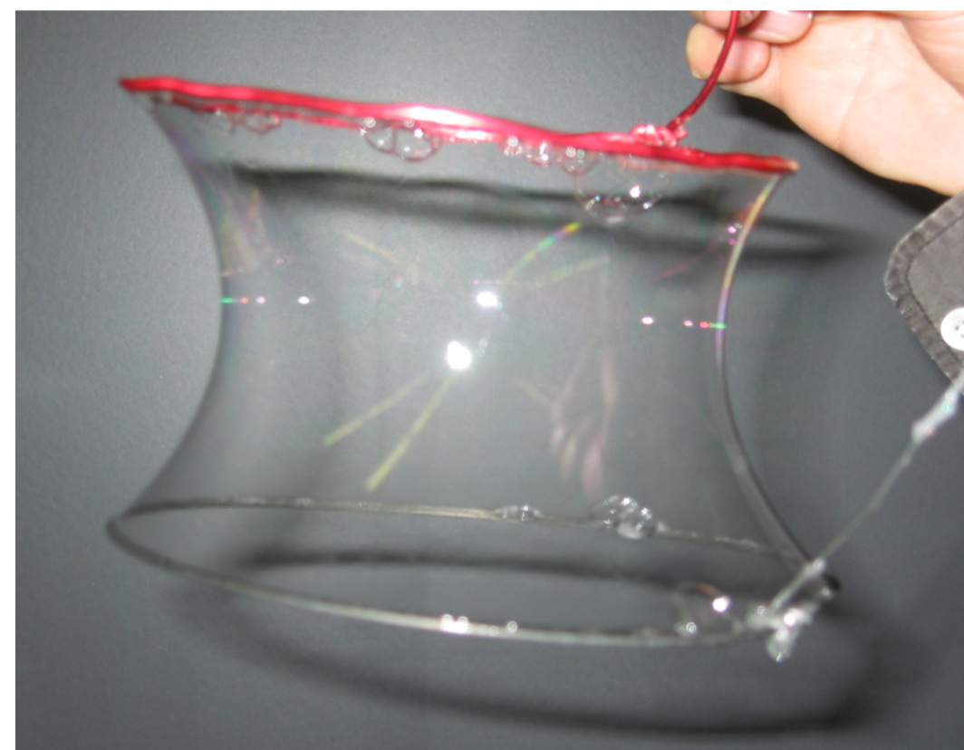
懸垂面 (カテナイド)
