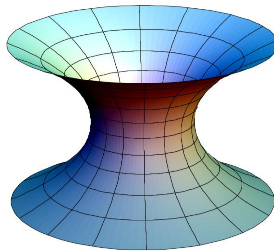
極小曲面の例
