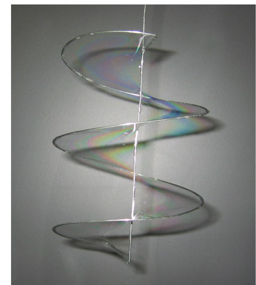
常螺旋面 (ヘリコイド)
