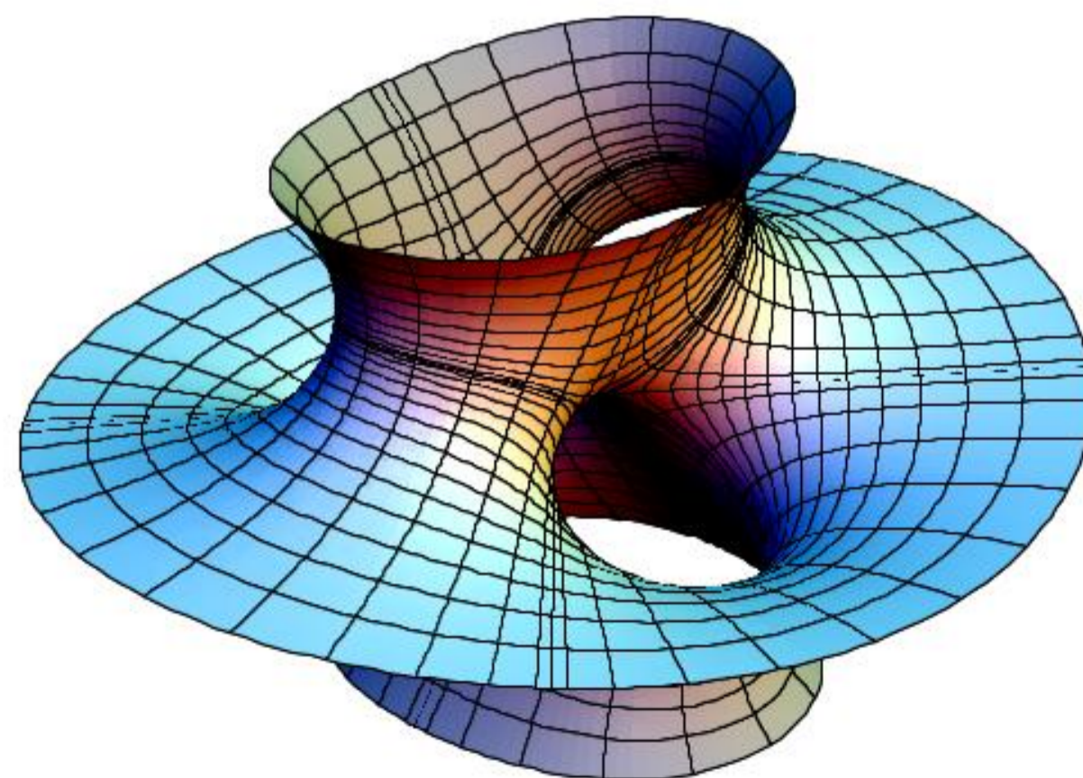
Costaの極小曲面
