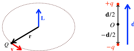
図 10: 左: 円運動する荷電粒子。右: 電気双極子。
