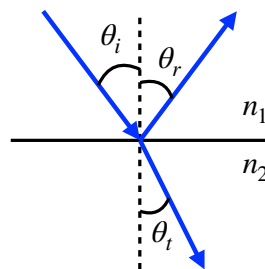
図 28: 媒質の境界での光の反射と屈折。
