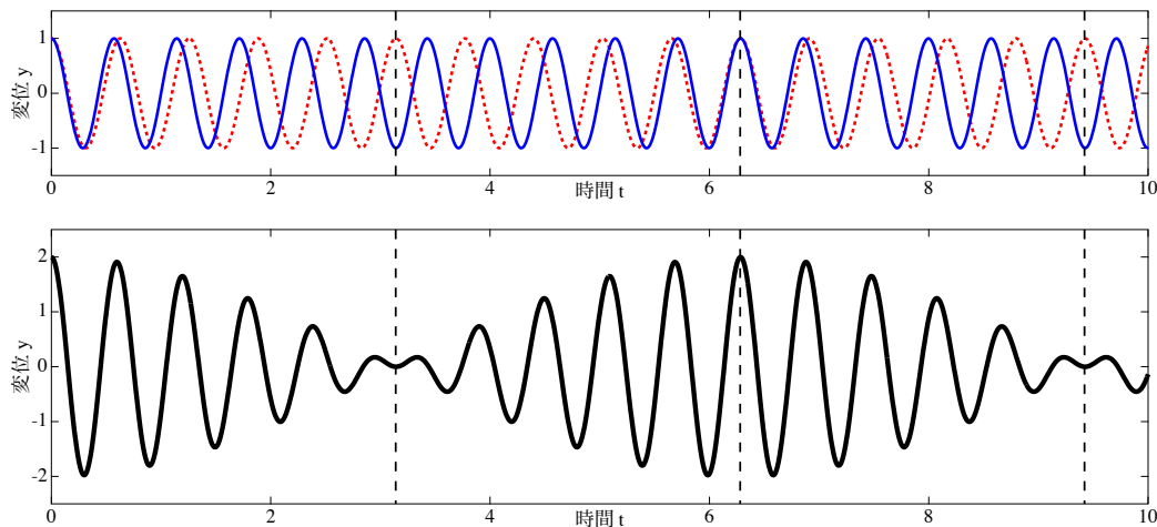
図 29: 波の重ね合わせ。上： y = \cos(11t) (実線) と y = \cos(10t) (点線) のグラフ。下： y = \cos(11t) + \cos(10t) のグラフ。縦の波線は t = n\pi/(2\omega) = n\pi ( \omega = 1/2 ) を表す。
