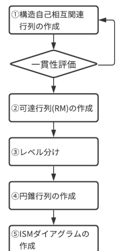
図-1 ISM 法のフロー
