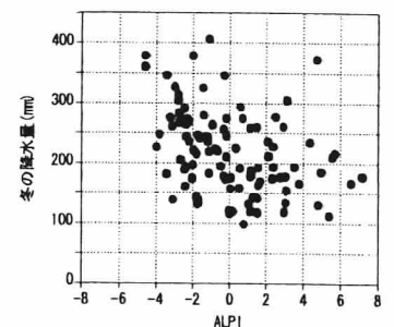
図-2 ALPI と冬の降水量の散布図
