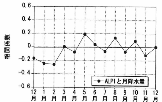
図-1 ALPI と月降水量の相互相関関係
