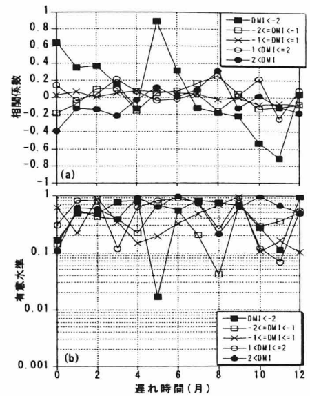
図-3 カテゴリー化した DMI と基準化月降水量の(a)相互相関数(b)有意水準
