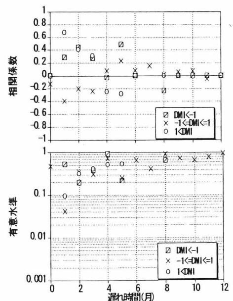
図-5 カテゴリー化した DMI と基準化した冬の降水量との(a)相互相関関数(b)有意水準
