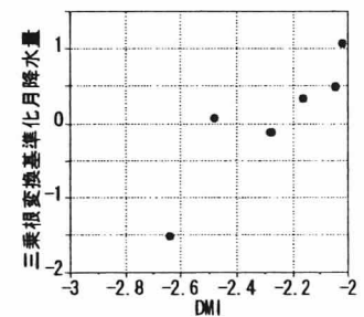
図-4 DMI のカテゴリー① (DMI < -2)における τ=5 ヶ月の散布図
