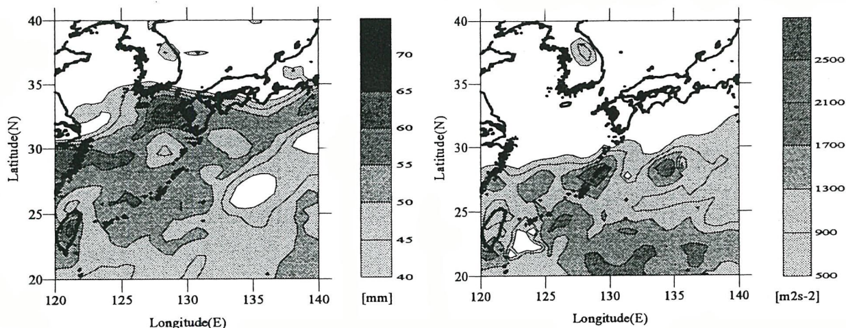
可降水量の分布
