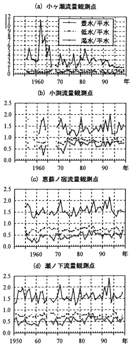
図-5 各流量観測点における平水流量で基準化した流況変動時系列
