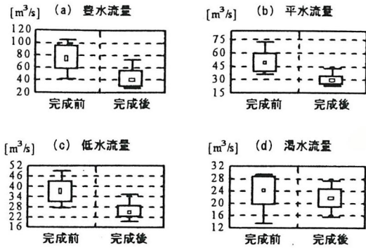
図-3 小湊流量観測点における下笠・松原ダム完成前後での流況比較箱ヒゲ図
