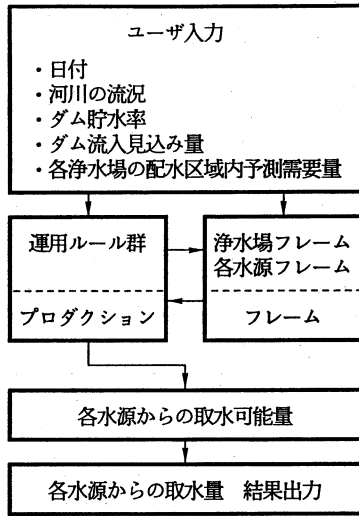
図-4 エキスパートシステムの構成
