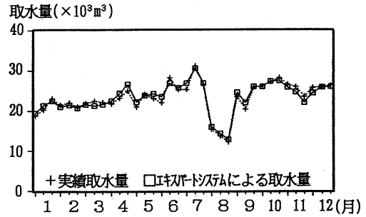
図-9 P 4 浄水場における取水量
