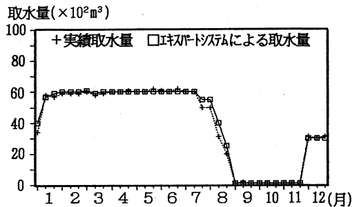
図-10 P 5 浄水場における取水量
