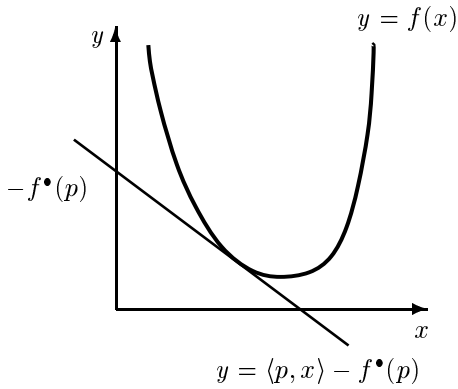
図 2: 共役関数 (Fenchel-Legendre 変換)
