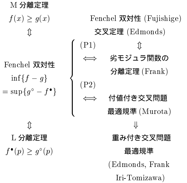
図 3: 双対定理の関係 ( f は M 凸関数, g は M 凹関数)
