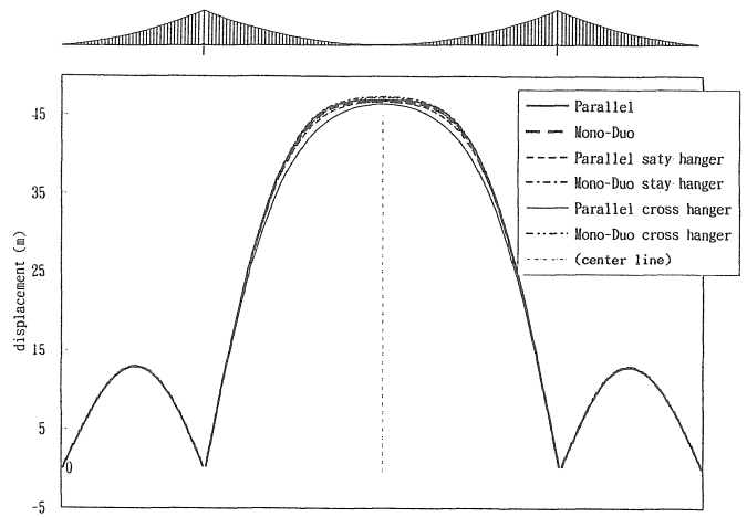
図-6.6 設計風荷重載荷時の補剛桁の橋軸直角方向変位
