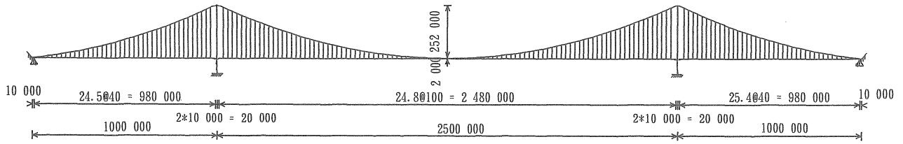
図-4.1 超長大吊橋の試設計例の一般図
