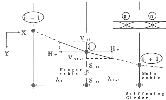
図-3.2 X-Y平面における作用力
