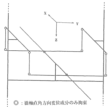
図-4.5 ウィンドシュアのモデル化
