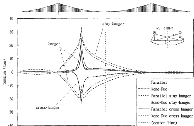
図-6.3 ハンガー、および、補助ハンガーの張力の影響線(ねじり荷重)
