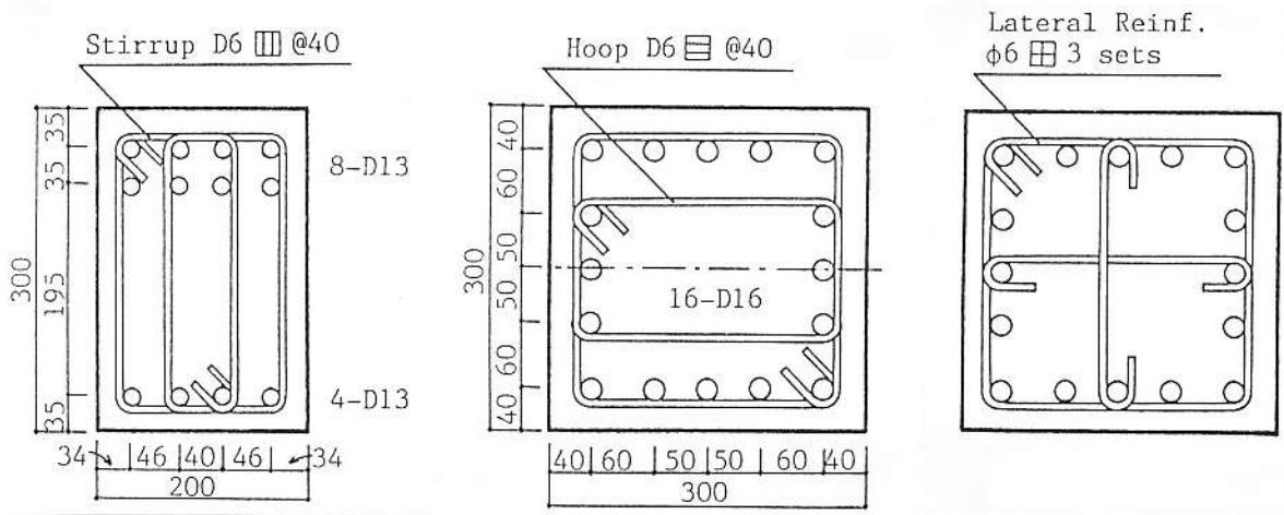
(b) 梁断面
