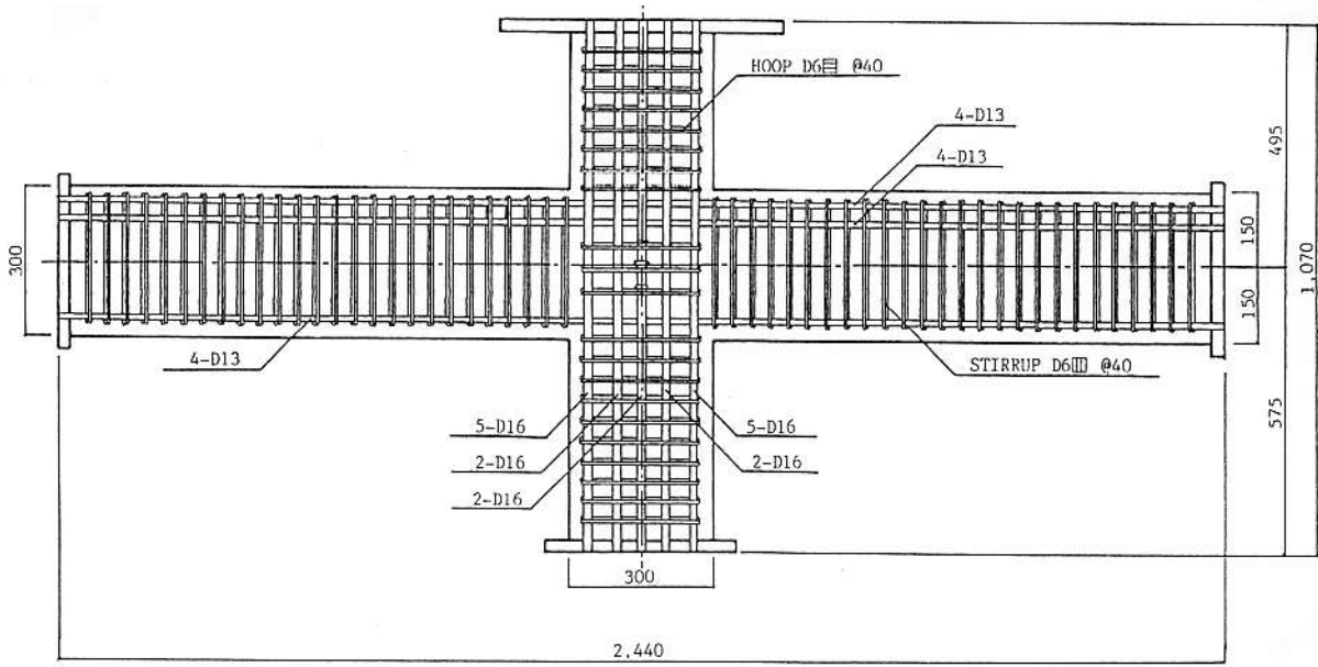
(a) 立面
