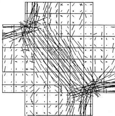
(c) 軸力 3 倍
