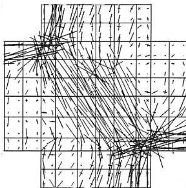
(e) 軸力 5 倍
