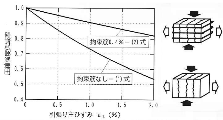
図6.1.5-2 直方体コンクリートの圧縮強度低減率（既往の実験結果）
