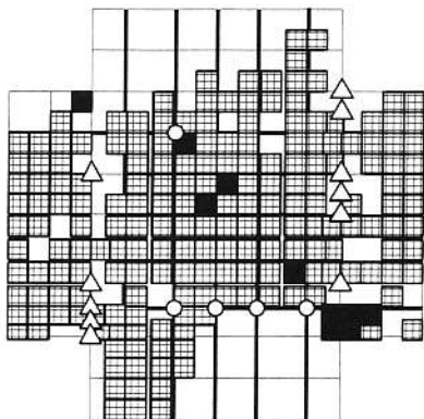
(e) 軸力 5 倍
