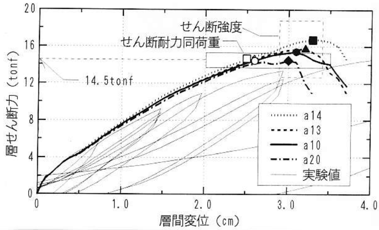
図6.1.5-6 層せん断力－層間変位関係 ～接合部横補強筋の量および強度を変数とした解析～
