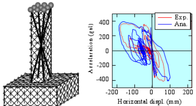
図3 三次元格子モデルによる二方向加力を受ける柱の解析
