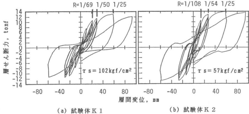
図5 層せん断力-層間変位関係
