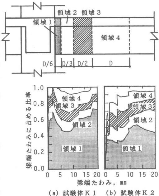
図7 梁局部回転が梁端たわみに占める割合
